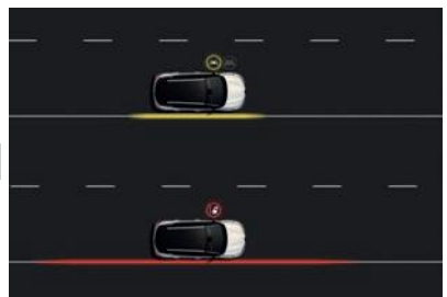
Sistem de asistență pentru menținerea benzii de rulare (LKA) și Sistem de avertizare la părăsirea involuntară a benzii de rulare (LDW)
